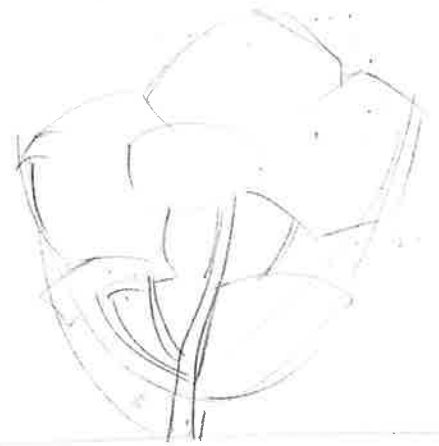
SESSILE OAK
