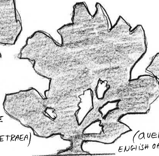
OAK CHÔNE
